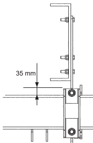
Illustration 28. Un espace d'au moins 35 mm est nécessaire pour le support de cadre entre le cadre du véhicule et l'ossature de l'élèveur
