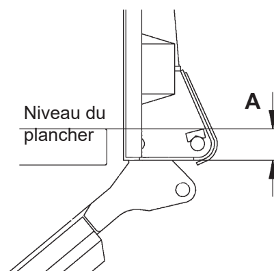
Illustration 35. Contrôle de la position par rapport à la traverse arrière du véhicule
