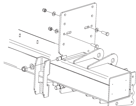
Illustration 27. Fixation du profilé en U avec ses rondelles et écrous
