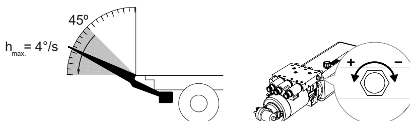
Illustration 53. Réglage de la vitesse de givrage vers le bas dans la plage de travail (à partir de 45° vers le bas)
