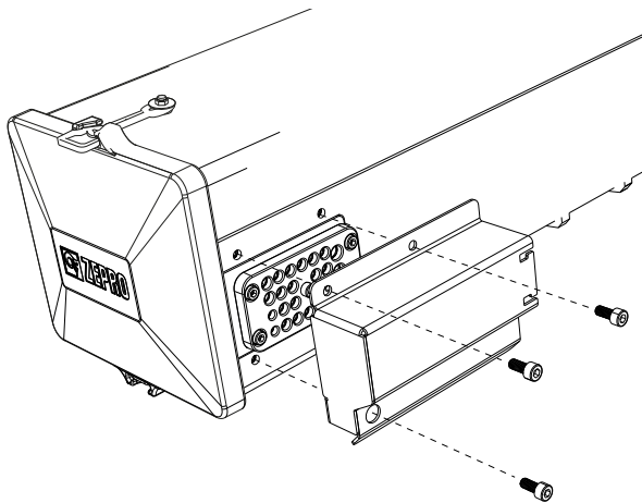
Illustration 73. Capot de protection du presse-étoupe maintenu par trois vis
