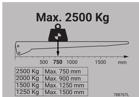
Illustration 84. Le diagramme de charge pour la capacité de charge 2500 kg, distance du centre de gravité 750 mm.
