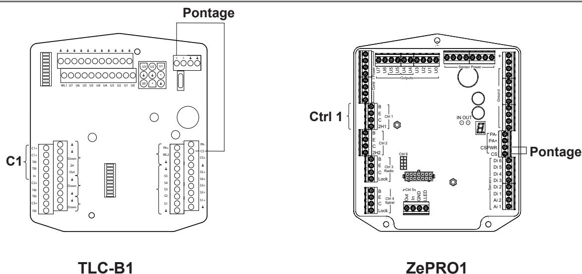
Illustration 23. Raccordement temporaire
