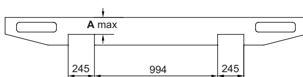
Illustration 16. ZDK 250
