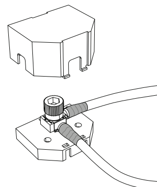
Illustration 81. Boîte à fusibles avec couvercle de protection
