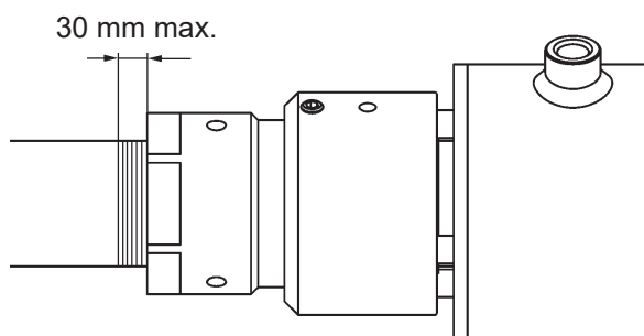
Illustration 40. Réglage de l'angle d'inclinaison
