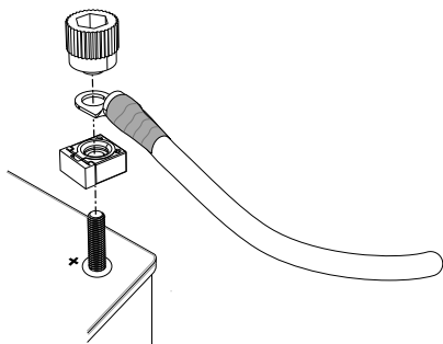
Illustration 67. Connexion au pôle plus de la batterie
