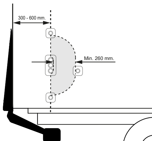
Illustration 59. Installation de l'actionneur CD 1 pour une utilisation à deux mains.
