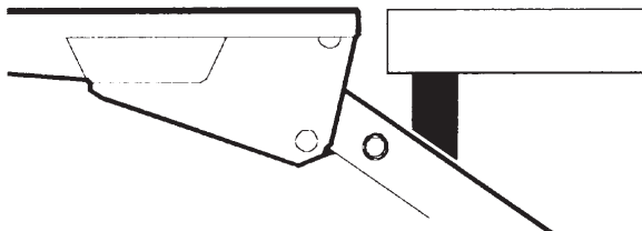
Illustration 45. Placez les butées d'arrêt entre les bras de levage et la traverse arrière du plancher
