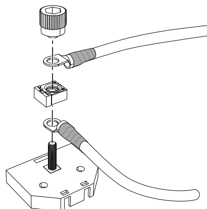
Illustration 68. Connexion à la boîte à fusibles
