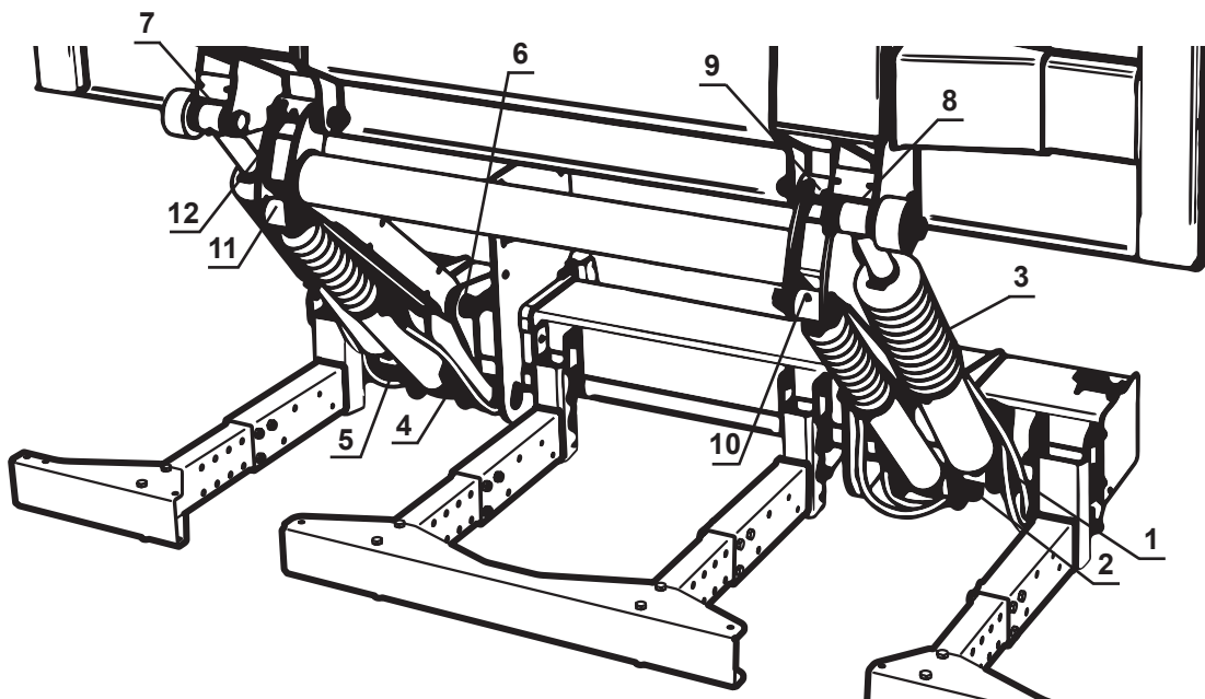
Illustration 82. Points de graissage
