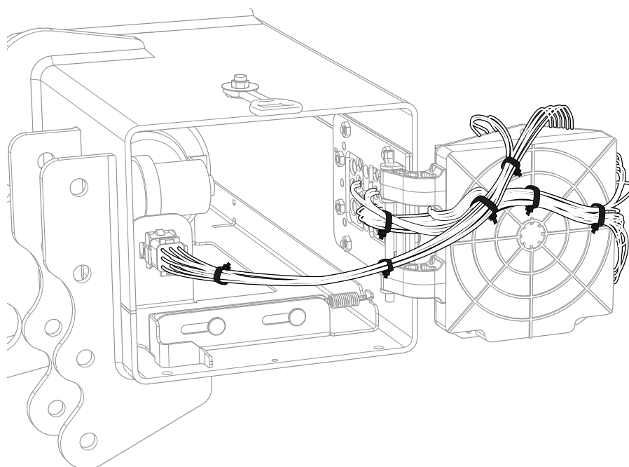
Illustration 76. Mise en place des faisceaux avec serre-câbles
