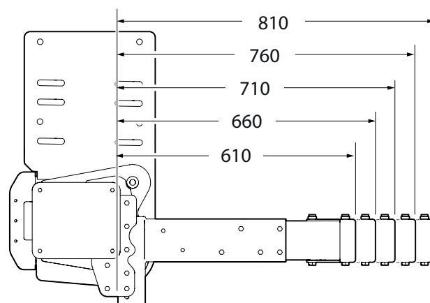
Illustration 48. La partie extérieure des supports peut être montée dans cinq positions différentes
