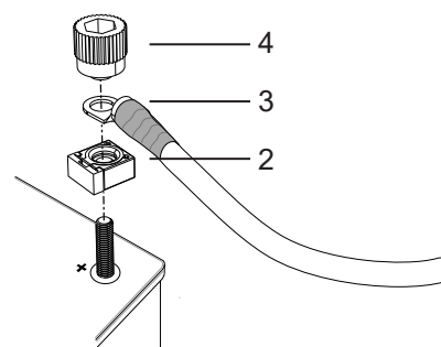
Illustration 78. Connexion au pôle plus de la batterie
