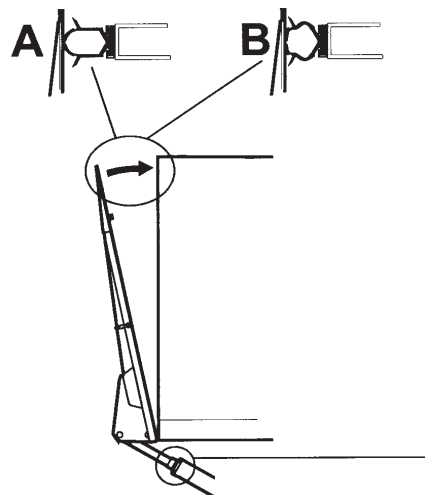
Illustration 37. Ajustement du contact contre la superstructure
