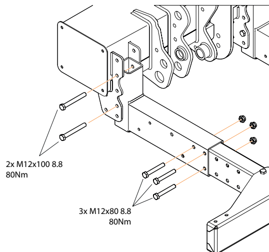
Illustration 49. Pose de la protection anti-encastrément
