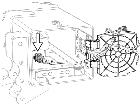
Illustration 19. Connecteur
