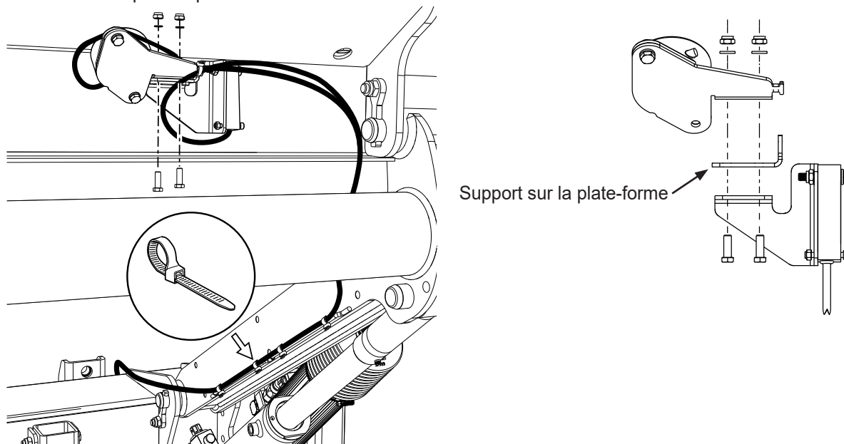
Illustration 56. Capteur d'angle de montage pour ouverture / fermeture automatique
