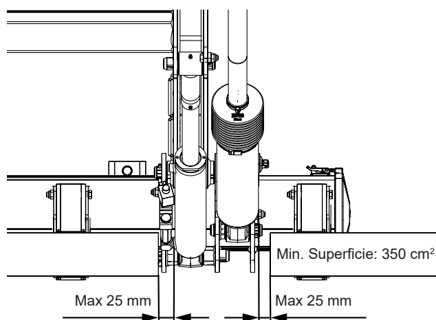
Illustration 10. Distances réglementaires
