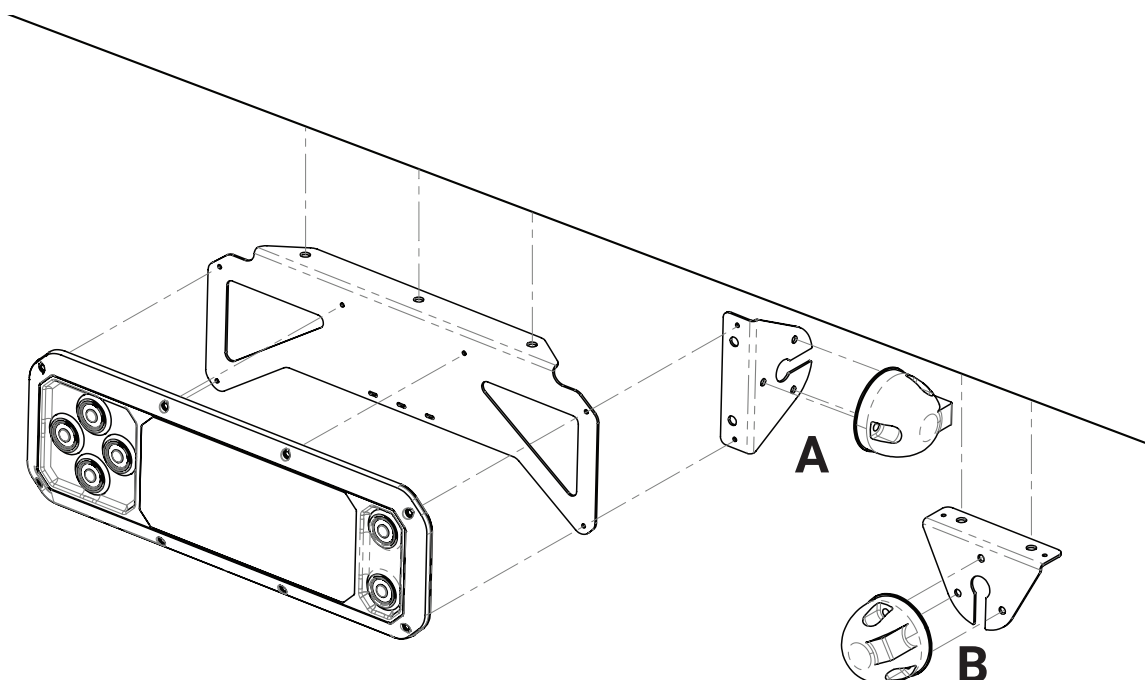
Illustration 63. Montage de l'actionneur portable CD 19 et contact pour l'actionneur portable
