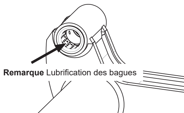
Illustration 31. Veillez à bien lubrifier les bagues métalliques
