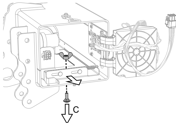
Illustration 20. Dégagement du groupe hydraulique
