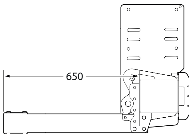
Illustration 14. ZDK 250 -155
