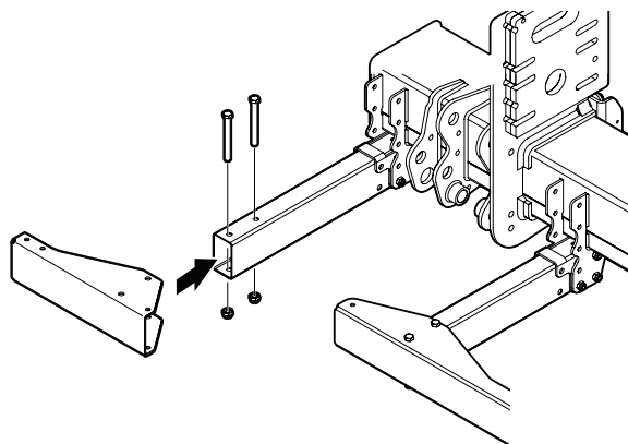
Illustration 51. Installation d'un profil en tôle intérieur
