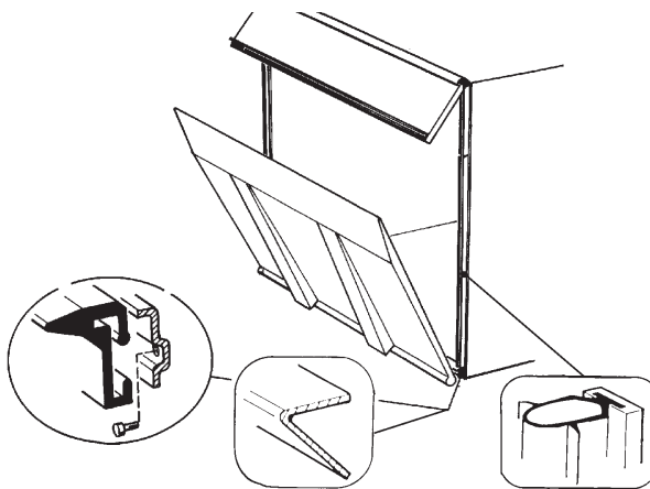
Illustration 46. Pose de la bande d'étanchéité
