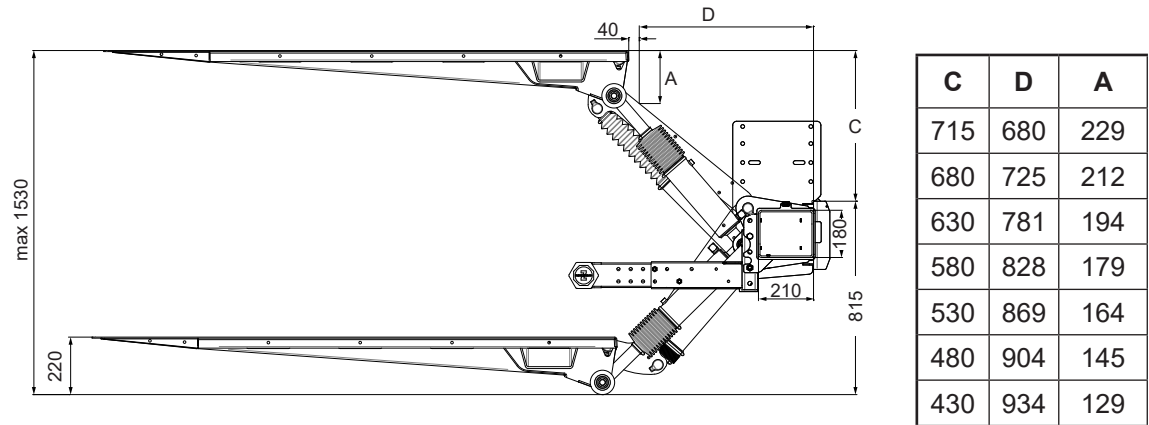
Illustration 12. ZDK 250-155
