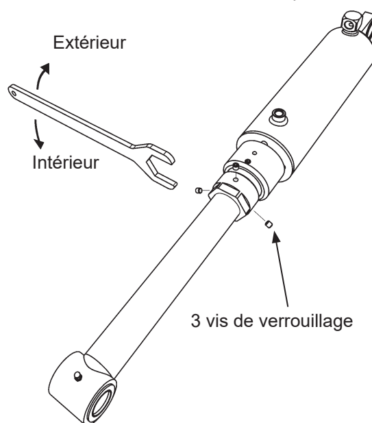
Illustration 36. Réglage de l'angle d'inclinaison
