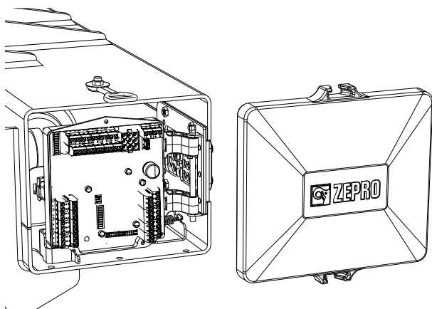
Illustration 17. Démontez le capuchon de protection
