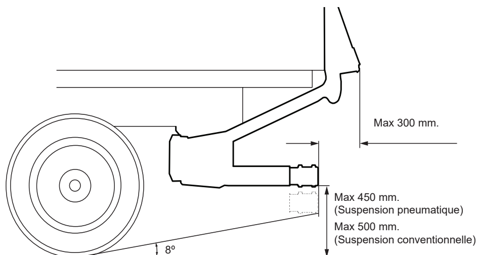
Illustration 8. Mesures réglementaires
