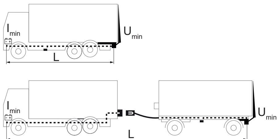
Illustration 66. Capacité de la batterie et définition de la longueur du câble d'alimentation principal et de terre
