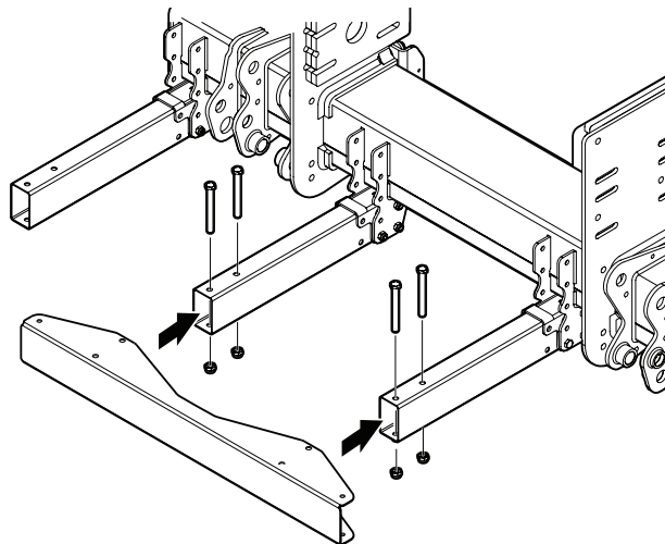
Illustration 51. Installation d'un profil en tôle intérieur
