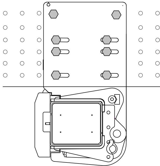
Illustration 30. Montage du support de cadre sur le cadre du véhicule avec pré-trous
