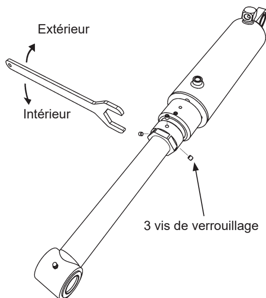
Illustration 38. Réglage de l'angle d'inclinaison
