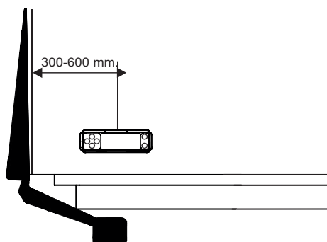
Illustration 61. Installation de l'actionneur
