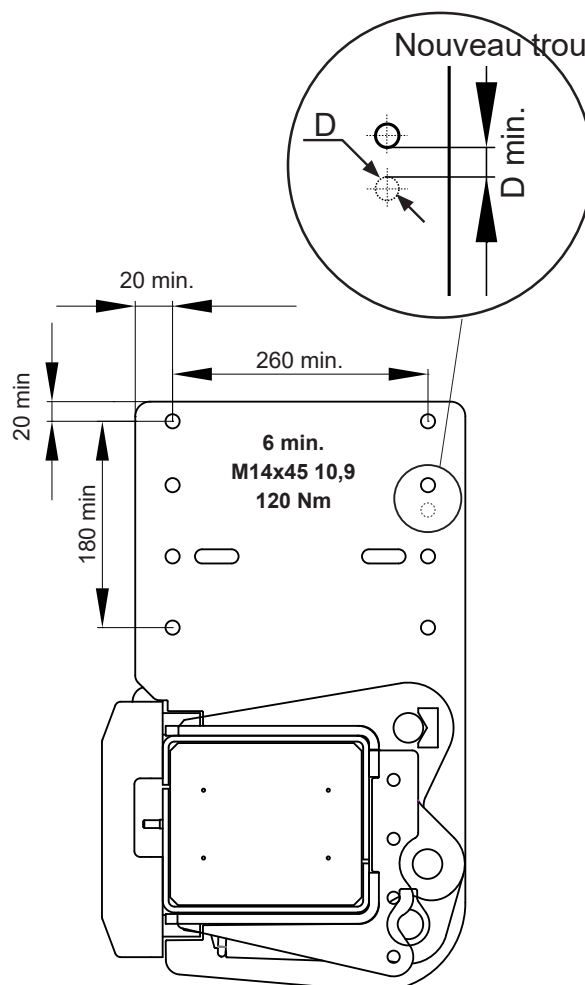
Illustration 29. Fixation du support de cadre avec au moins 6 boulons M14x45 10,9
