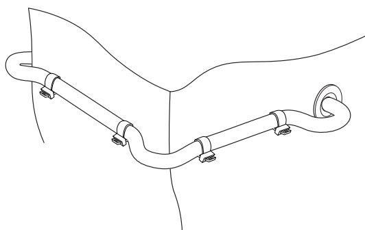
Illustration 64. Protégez le câble de toute arête vive et utilisez des presse-étoupes
