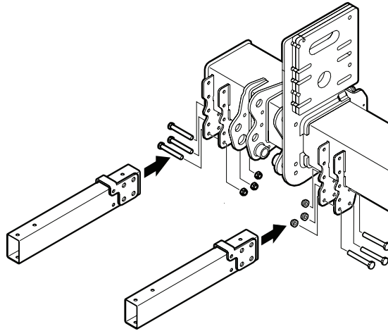
Illustration 50. Montage des supports sur le tube porteur
