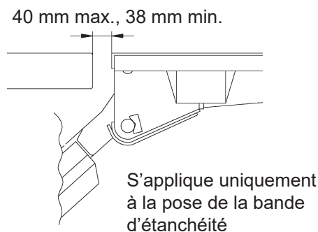
Illustration 35. Contrôle de la position par rapport à la traverse arrière du véhicule
