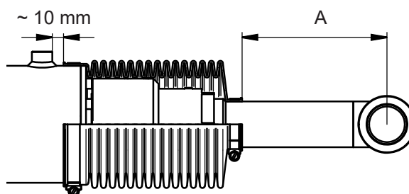
Illustration 41. Pose du manchon
