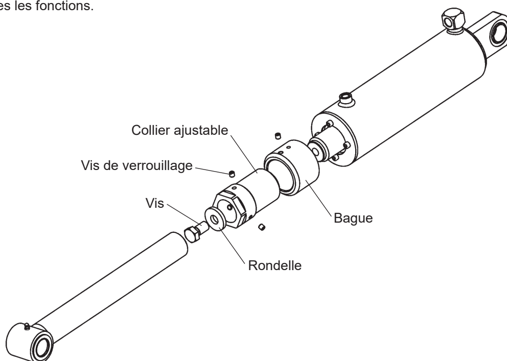
Illustration 44. Vérin d'inclinaison
