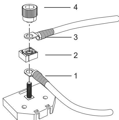
Illustration 77. Connexion à la boîte à fusibles
