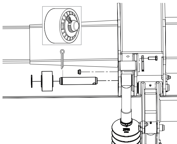
Illustration 39. Montage du vérin d'inclinaison sur la plate-forme
