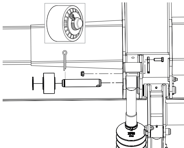
Illustration 33. Montage du vérin d'inclinaison sur la plate-forme
