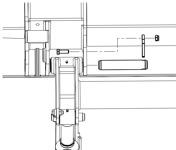
Illustration 32. Montage de la plate-forme sur les bras
